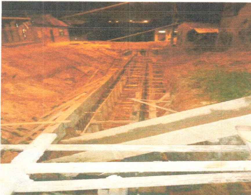
VISTA FOTOGRÁFICA N° 06 – VACEADO DE LOSA TECHO CANAL.
