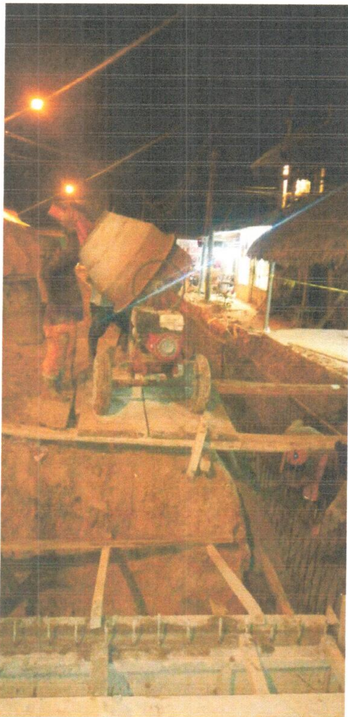
VISTA FOTOGRÁFICA N° 08 – VACEADO DE MURO CANAL EN CALLE CASTAÑAL
